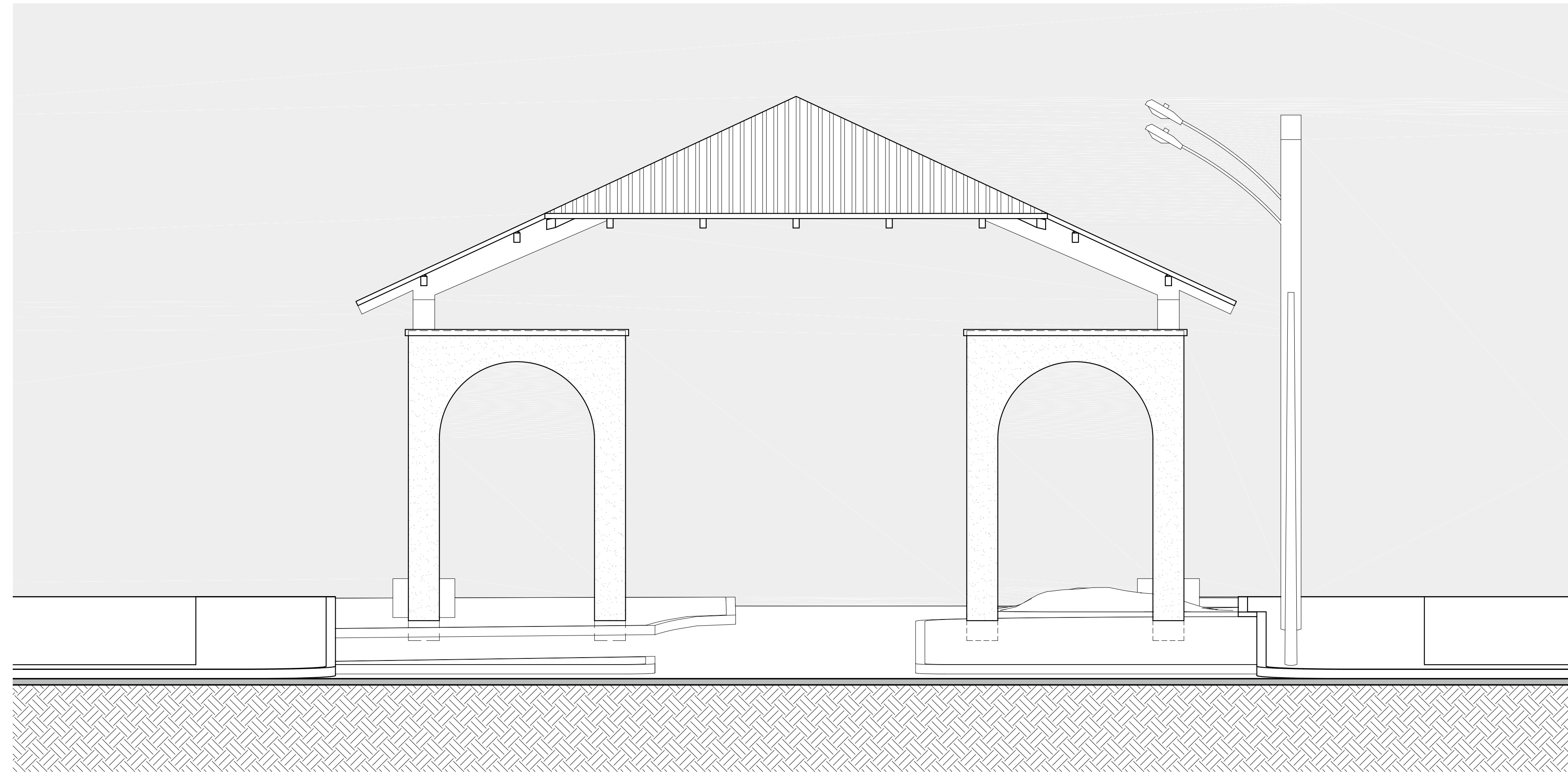
01 FACHADA LESTE Escala 1:50
