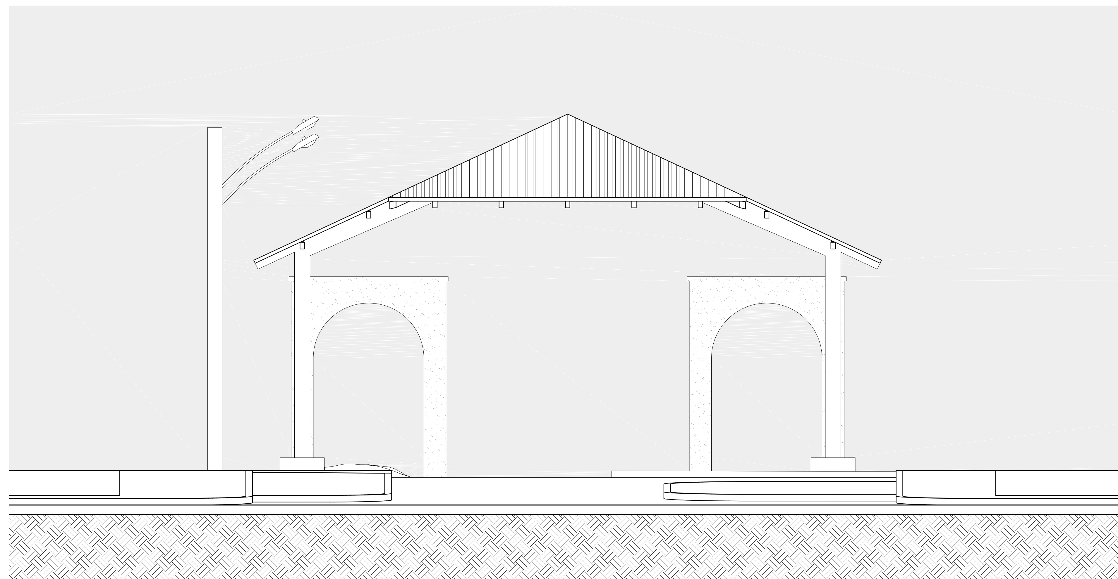
02 FACHADA OESTE Escala 1:50
