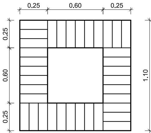
Planta Baixa
