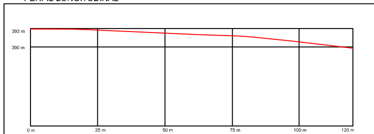
PERFIL LONGITUDINAL
