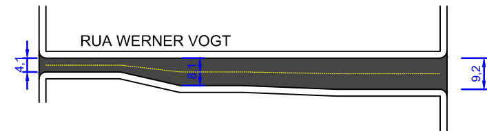
SEÇÃO TRANSVERSAL
