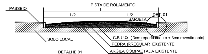
SEÇÃO TRANSVERSAL TÍPICA Esc Indet.
