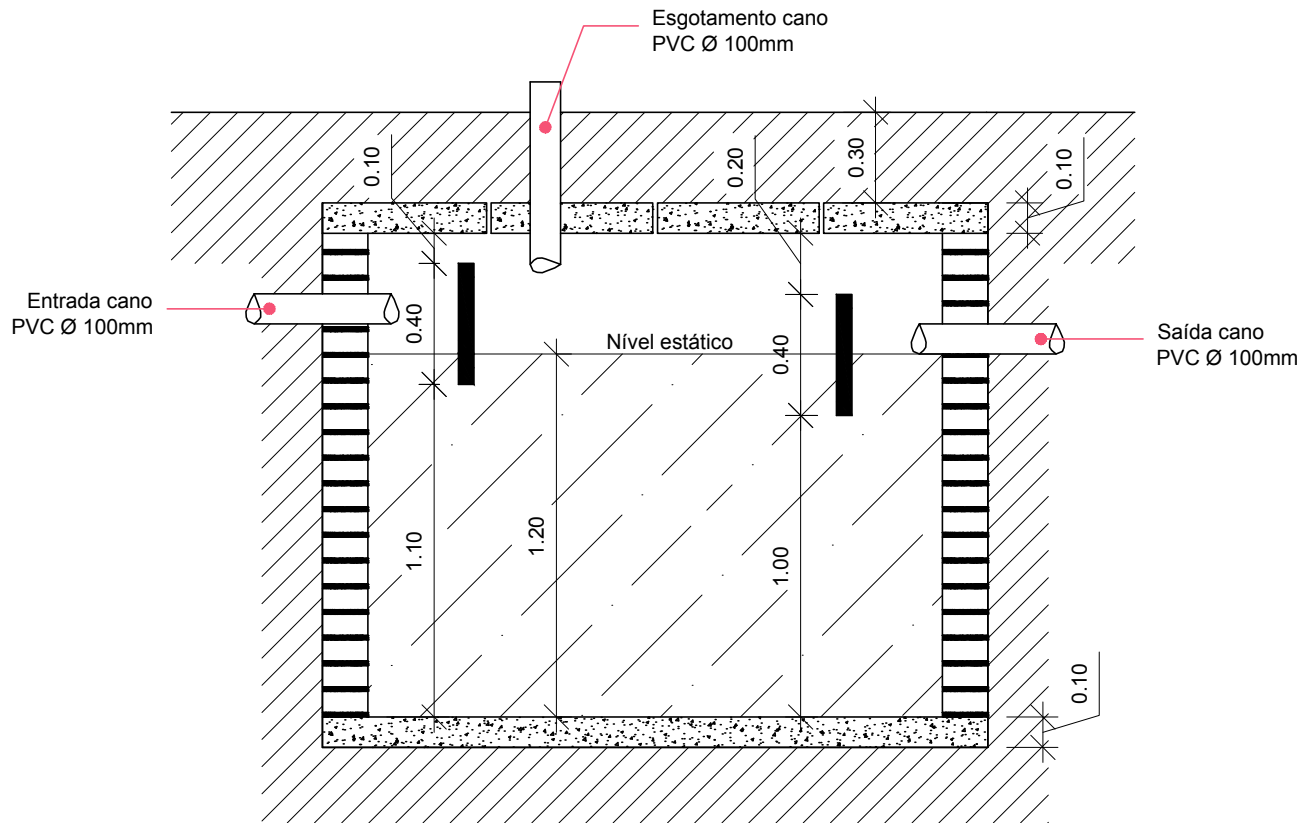
CORTE X. X'
