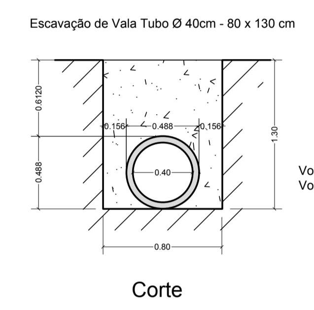
04 DETALHE DA ESCAVAÇÃO DAS VALAS ESCALA 1:25
