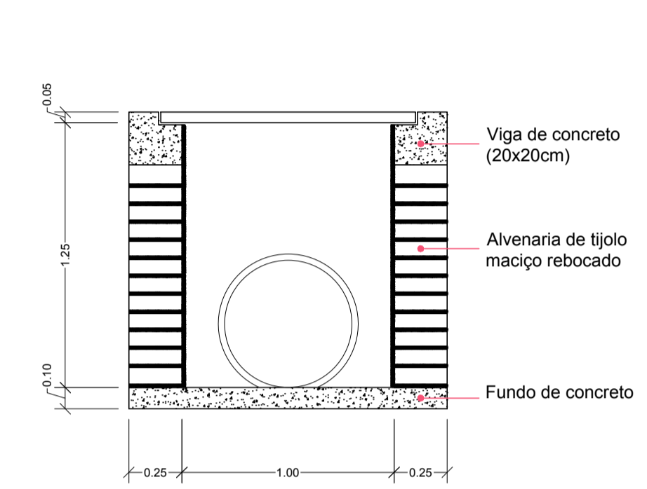
02 DETALHE DA CAIXA COLETORA 2 ESCALA 1:25
