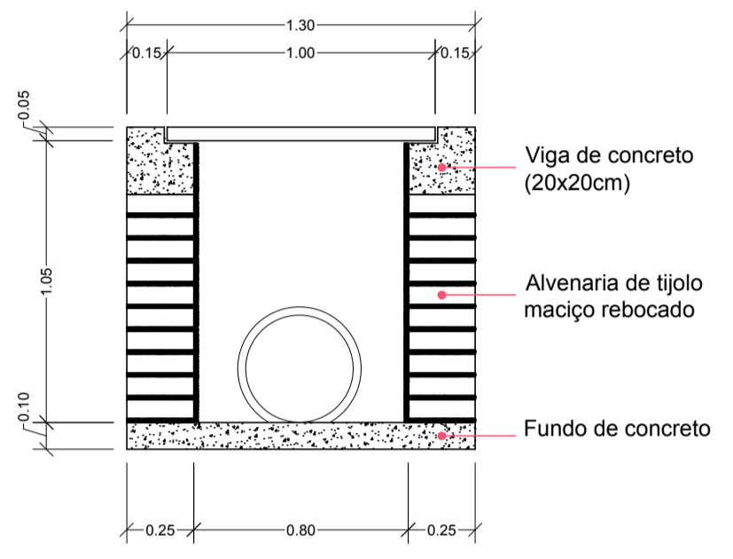
01 DETALHE DA CAIXA COLETORA 1 ESCALA 1:25
