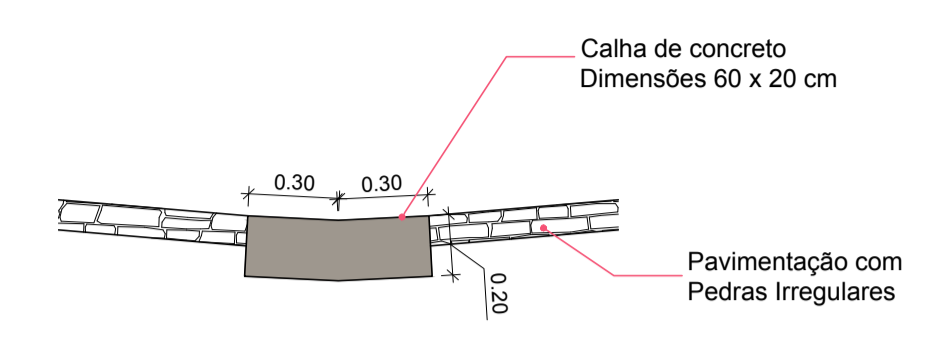
03 DETALHE DA CALHA ESCALA 1:25
