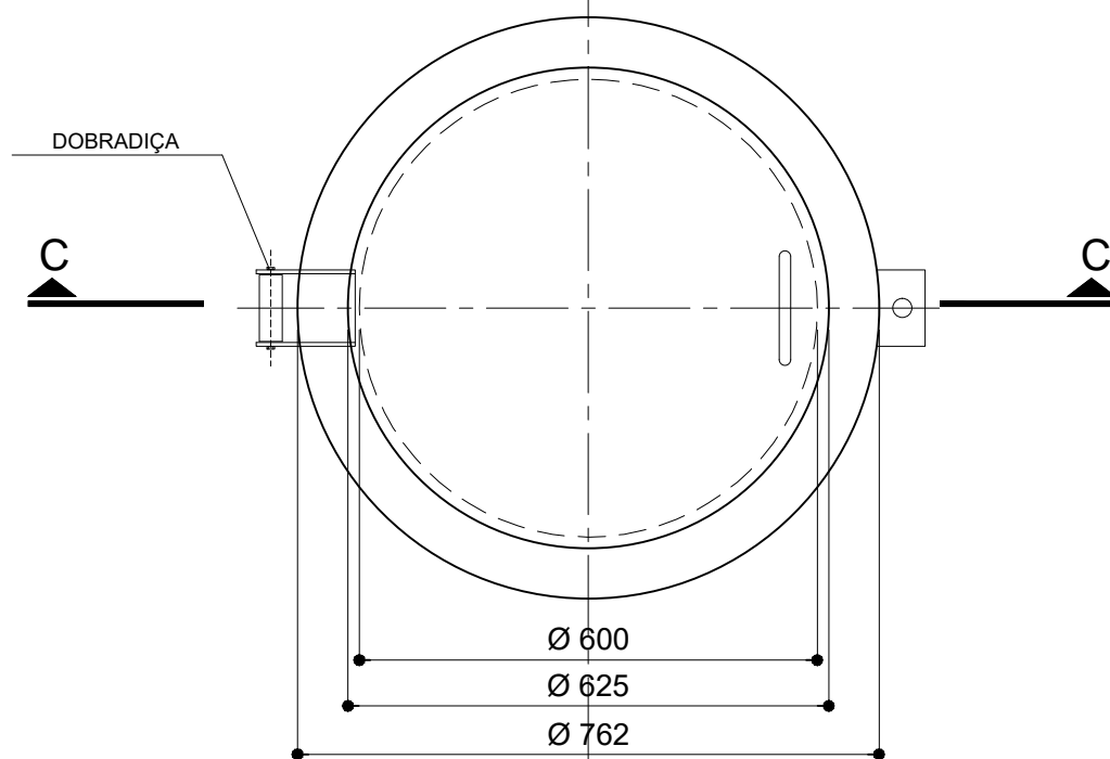
DET. TAMPA DE INSPEÇÃO SUPERIOR
