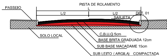
SEÇÃO TRANSVERSAL TÍPICA Esc. Ind.
