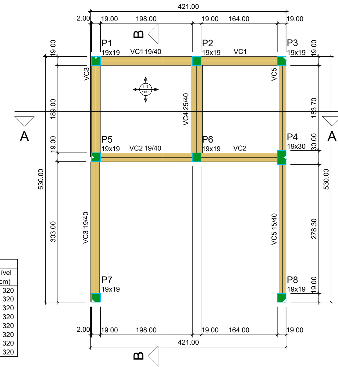
FORMA DO PAVIMENTO COBERTURA (NÍVEL 320) Esc.: 1:50
