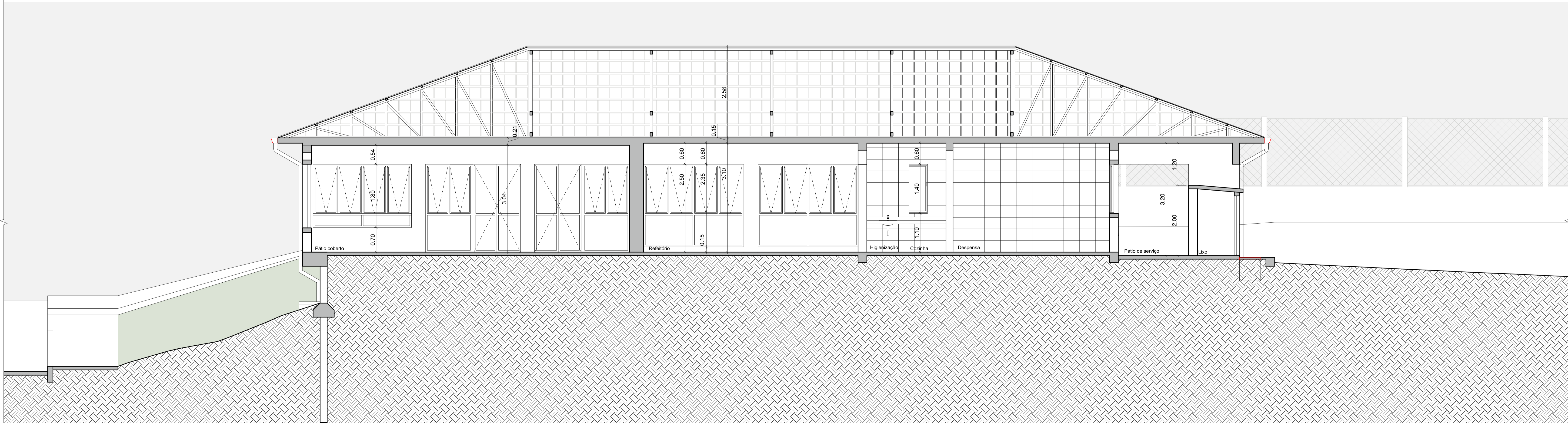
02 CORTE B.B' ESCALA 1:50
