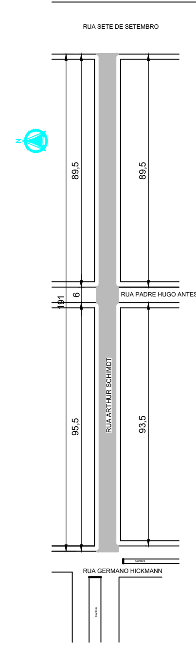
PLANTA BAIXA
