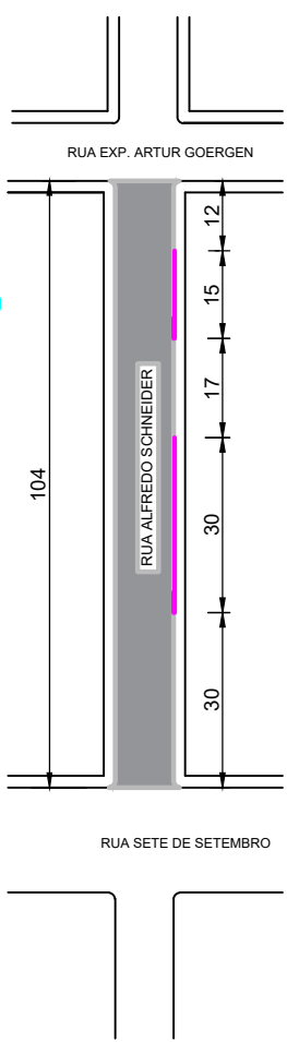
PLANTA BAIXA
