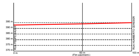
PERFIL LONGITUDINAL RUA OTTO RHUDEL
